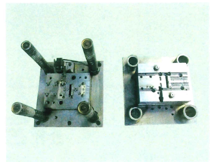
材質 SK85-A 板厚 t1.4 単発金型
