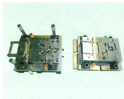
材質 SUS301-1/2H-CSP 板厚 t0.6 順送金型
