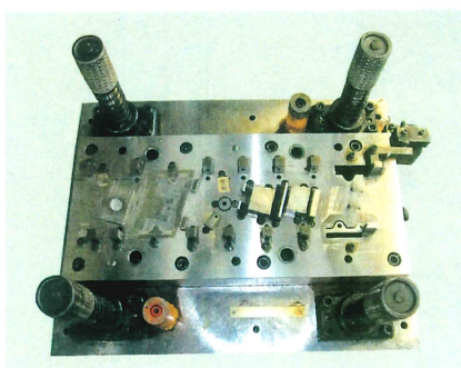
材質 SPCC 板厚 t2.3 順送金型
